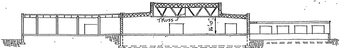
SECTION "A-A" SCALE: 1" = 50'
